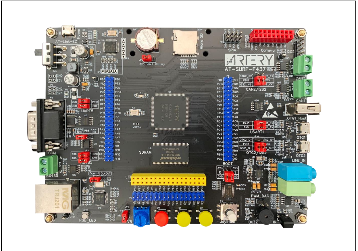
图 1. AT-START-F437 V1.0 开发板
